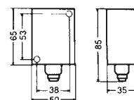
F 897 001 (Schutzart IP 65) (Protection class IP 65)
